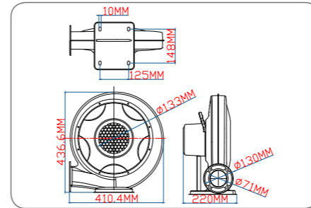
750W 铁机技术线图
