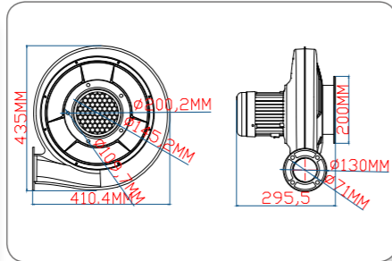
370W 喷砂设备铁机技术线图
