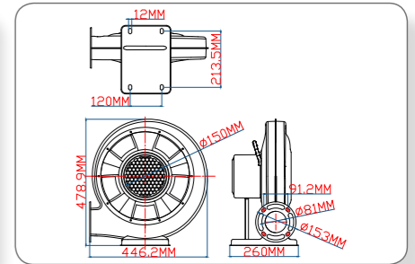
1100W 铁机技术线图
