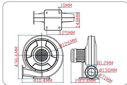
550W 厨具铁机技术线图
