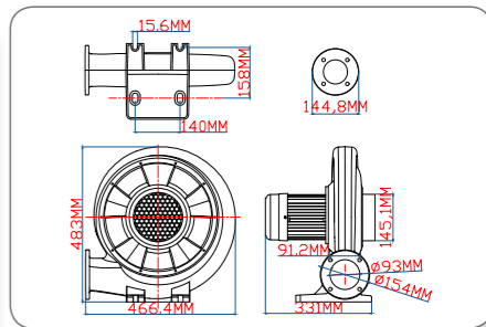
950W 激光雕刻风机技术线图
