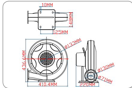
550W 铁机 A 款技术线图
