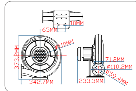
250W 厨具铁机技术线图
