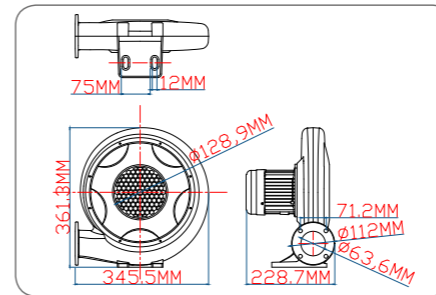
250W 厨具铝机技术线图
