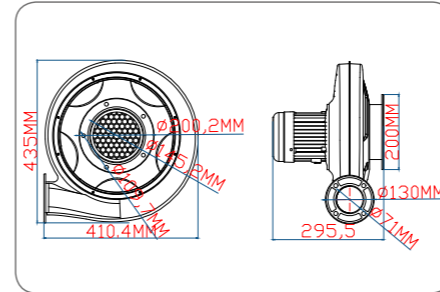
750W 喷砂铁机小款技术线图
