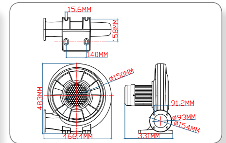
750W-950W 厨具铝机技术线图
