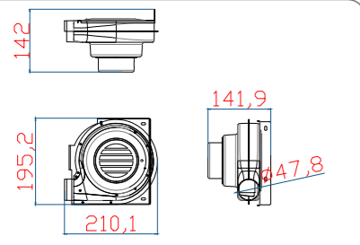
70W 节能机技术线图
