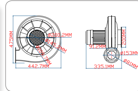
750W 喷砂设备铁机技术线图
