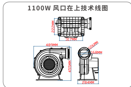
1100W-1500W 风口在上塑机
