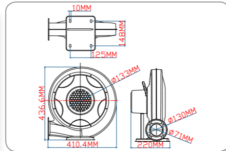
680W 铁机技术线图
