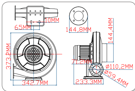
250W 激光雕刻风机技术线图
