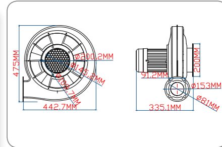
950W 喷砂设备铁机技术线图
