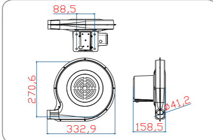
120W 菊花机技术线图
