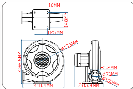
750W 厨具铁机 (小款) 技术线图
