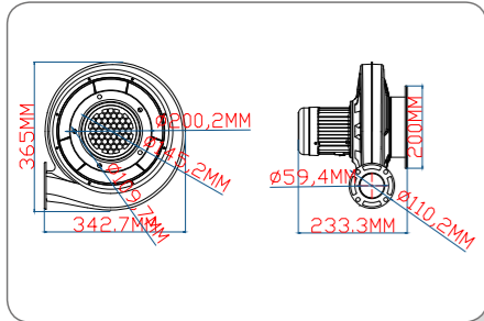
250W 喷砂设备铁机技术线图
