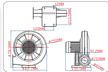
750W 厨具铁机技术线图
