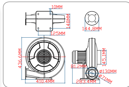
370W 激光雕刻风机技术线图
