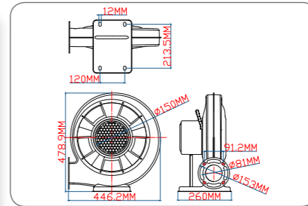
950W 铁机技术线图
