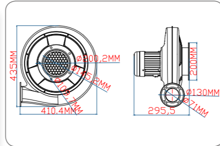
550W 喷砂设备铁机技术线图
