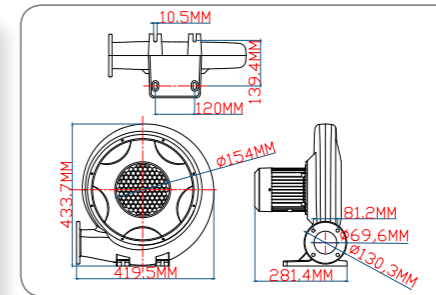
370W-550W 厨具铝机技术线图
