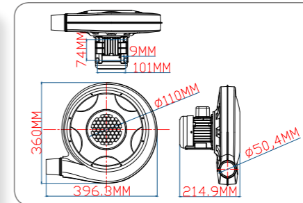
280W 厨具铁机技术线图
