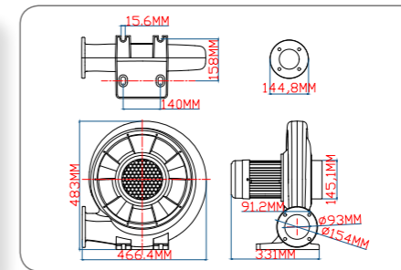
750W 激光雕刻风机技术线图
