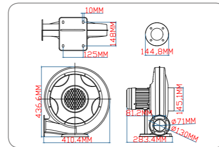
750W 小款激光雕刻风机技术线图
