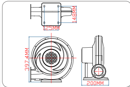
550W 铁机 C 款技术线图
