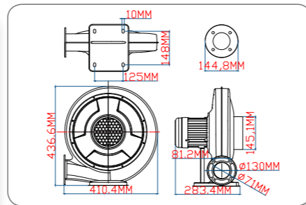
550W 激光雕刻风机技术线图
